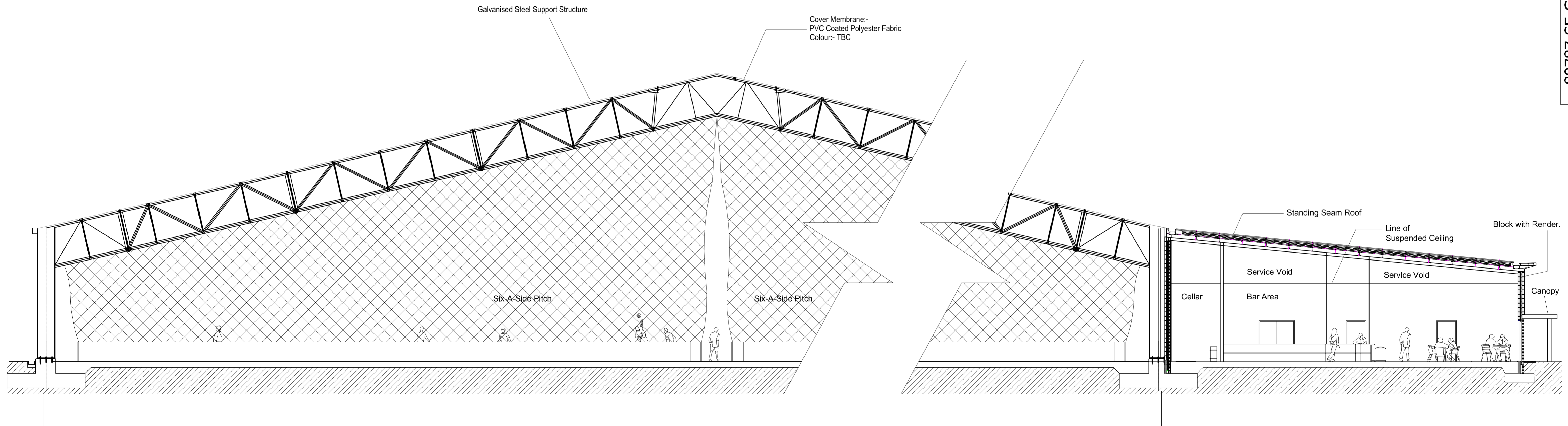
Section A-A 1:100
