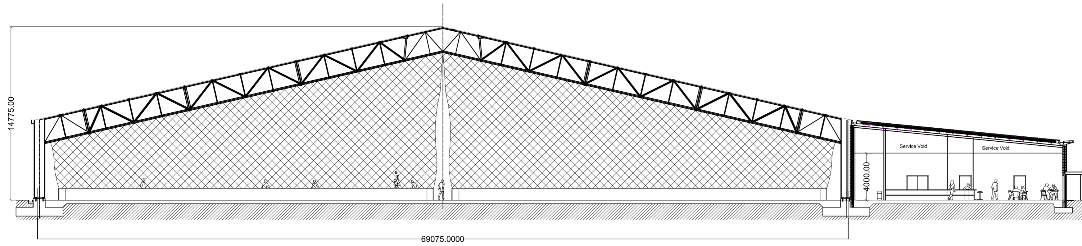
Section A-A 1:200
